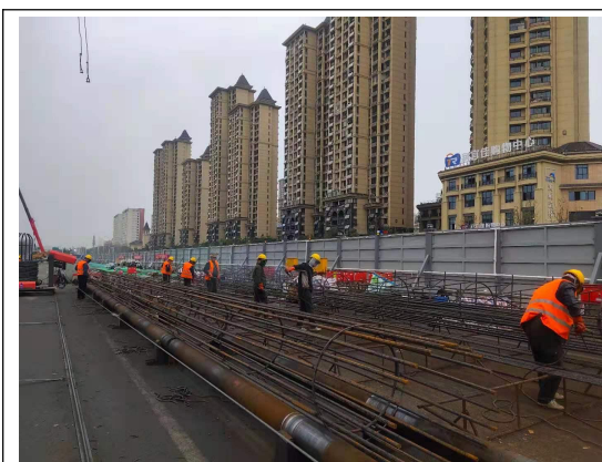
清潭路站钢筋笼加工
