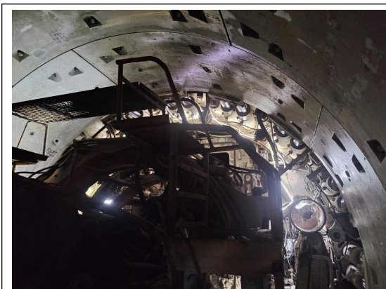
石门路站-耕耘路站区间左线盾构掘进施工
