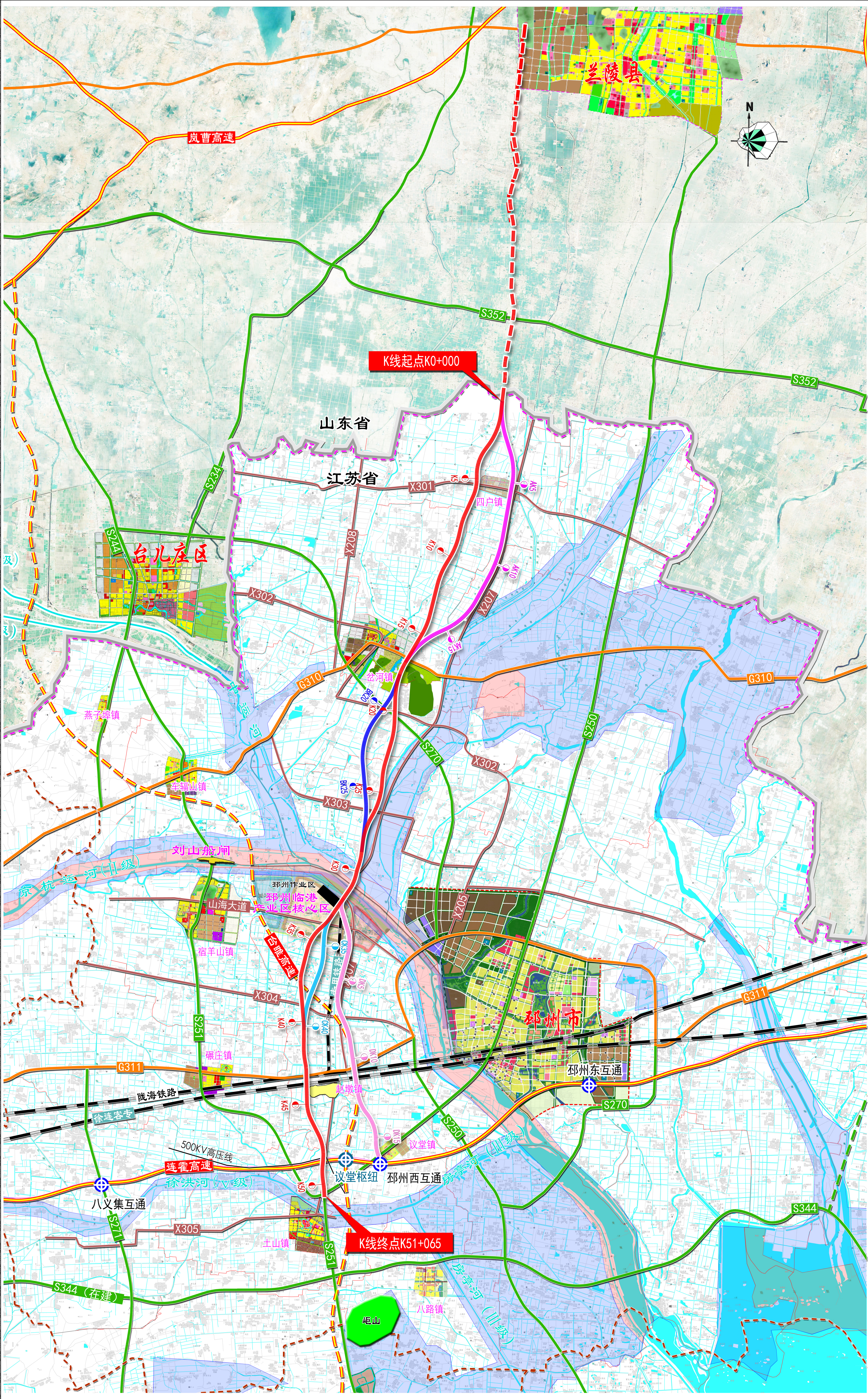
连霍高速公路邳州西互通连接线暨邳州疏港公路路线方案示意图
