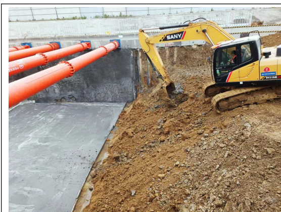
土方开挖及钢支撑架设--出入场线
