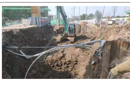
钟油坊路站雨污水管道开挖
