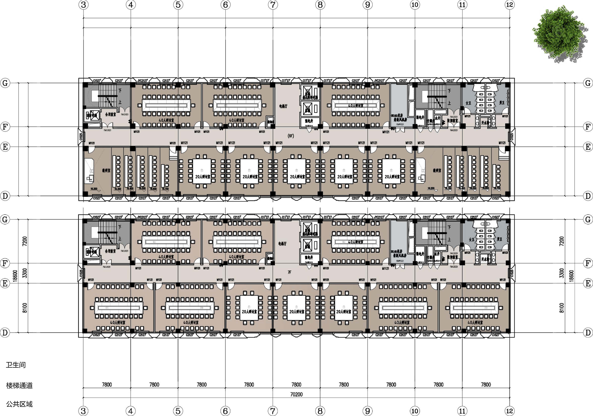
六-七层平面图
