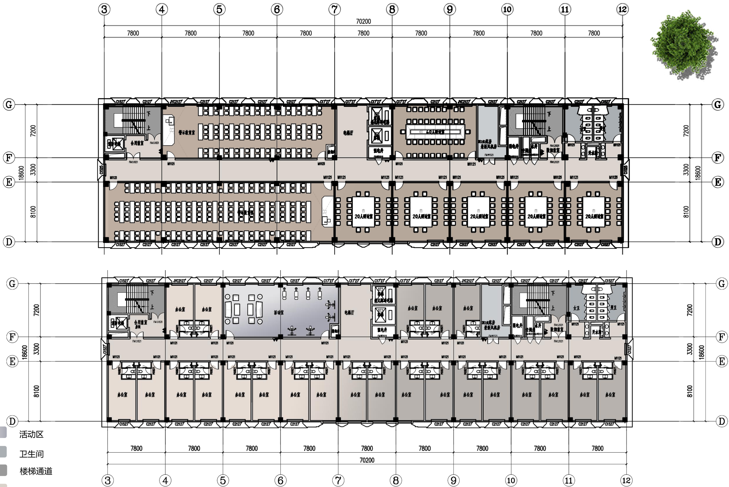
八-九层平面图
