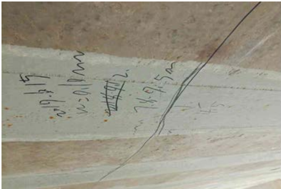
图 1-13 底板箱外面纵向裂缝
