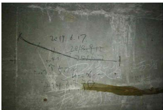
图 1-19 21#墩端横隔梁水平裂缝
