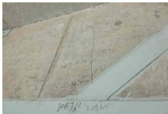
图 1-18 内侧腹板箱外面竖向裂缝
