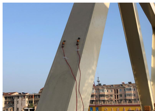
图 F1-1 传感器安装
