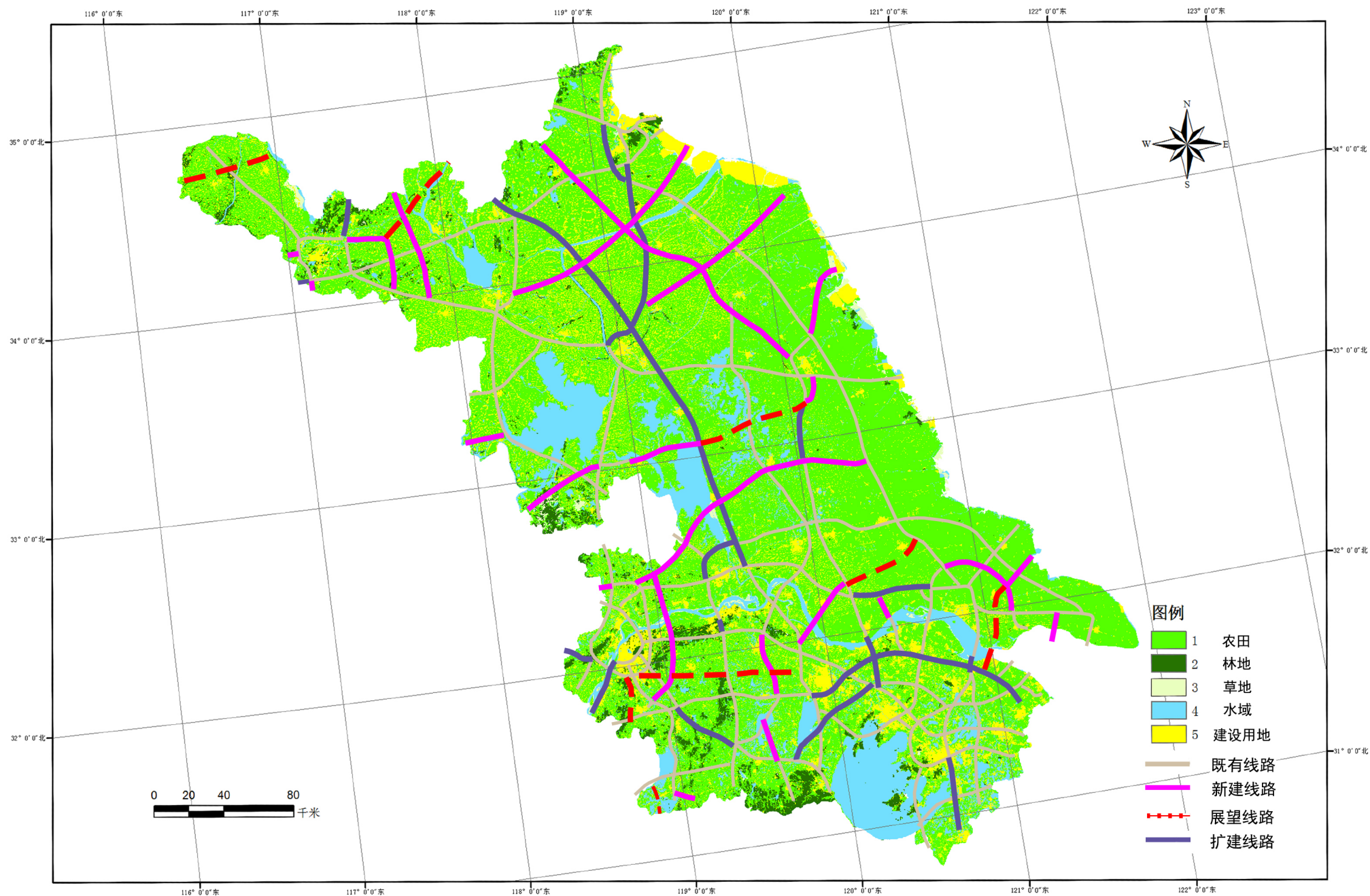
附图6 江苏省高速公路网与江苏省土地现状位置关系图
