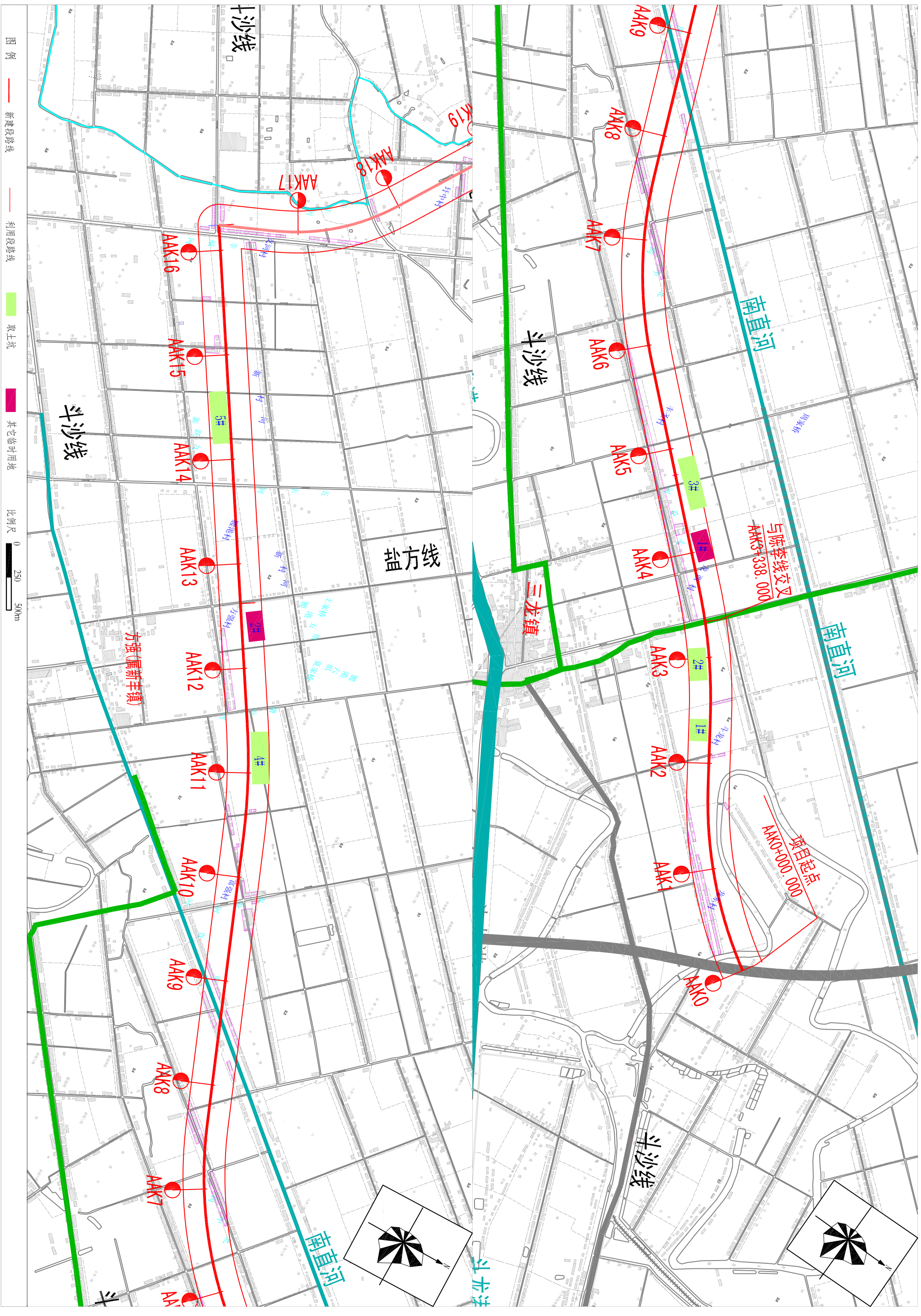
附图4 项目总平面布置图(1)
