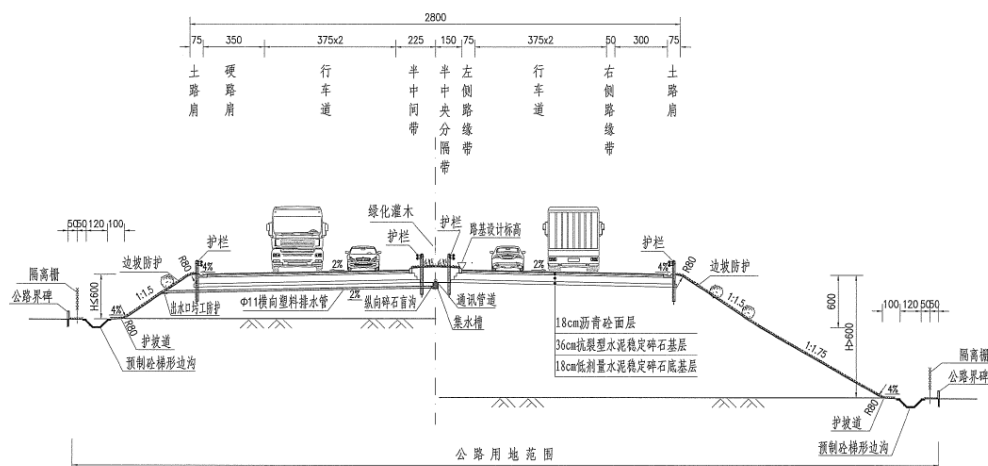
主线路基标准横断面
