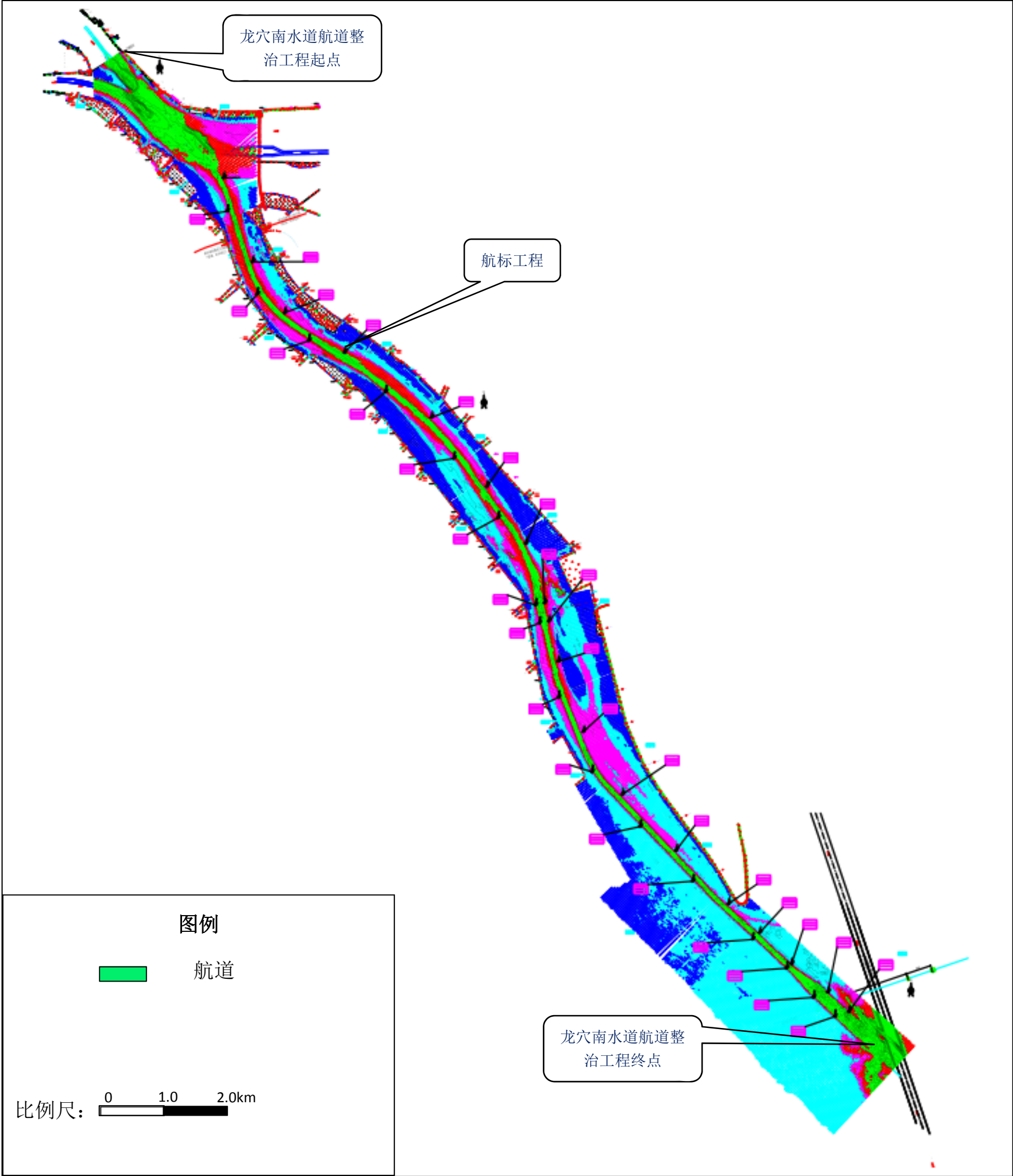
附图二：航道工程平面布置图
