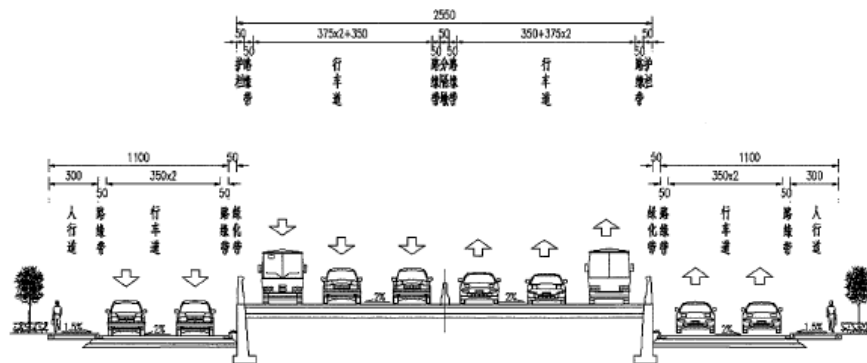
起点至高架桥桥头段道路标准横断面图
