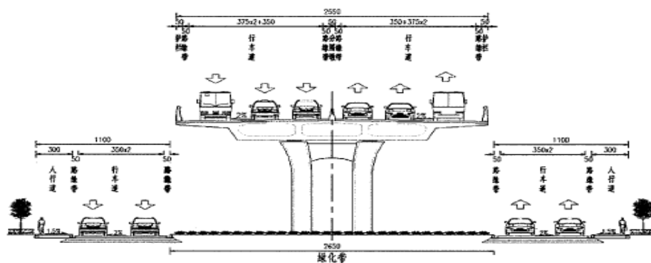
高架桥头至匝道起点段道路标准横断面图
