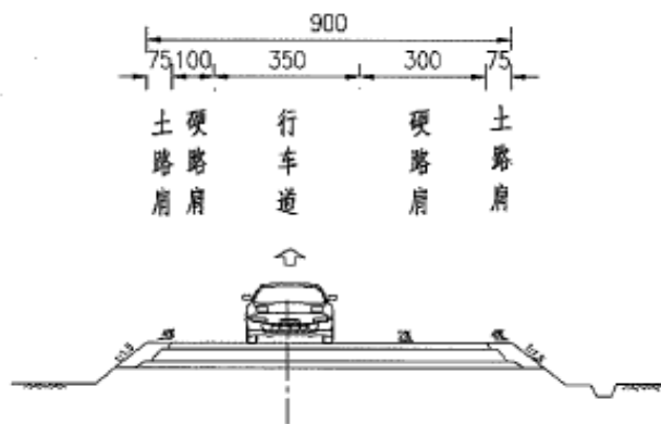
绕城公路入口 A 匝道路标准横断面图
