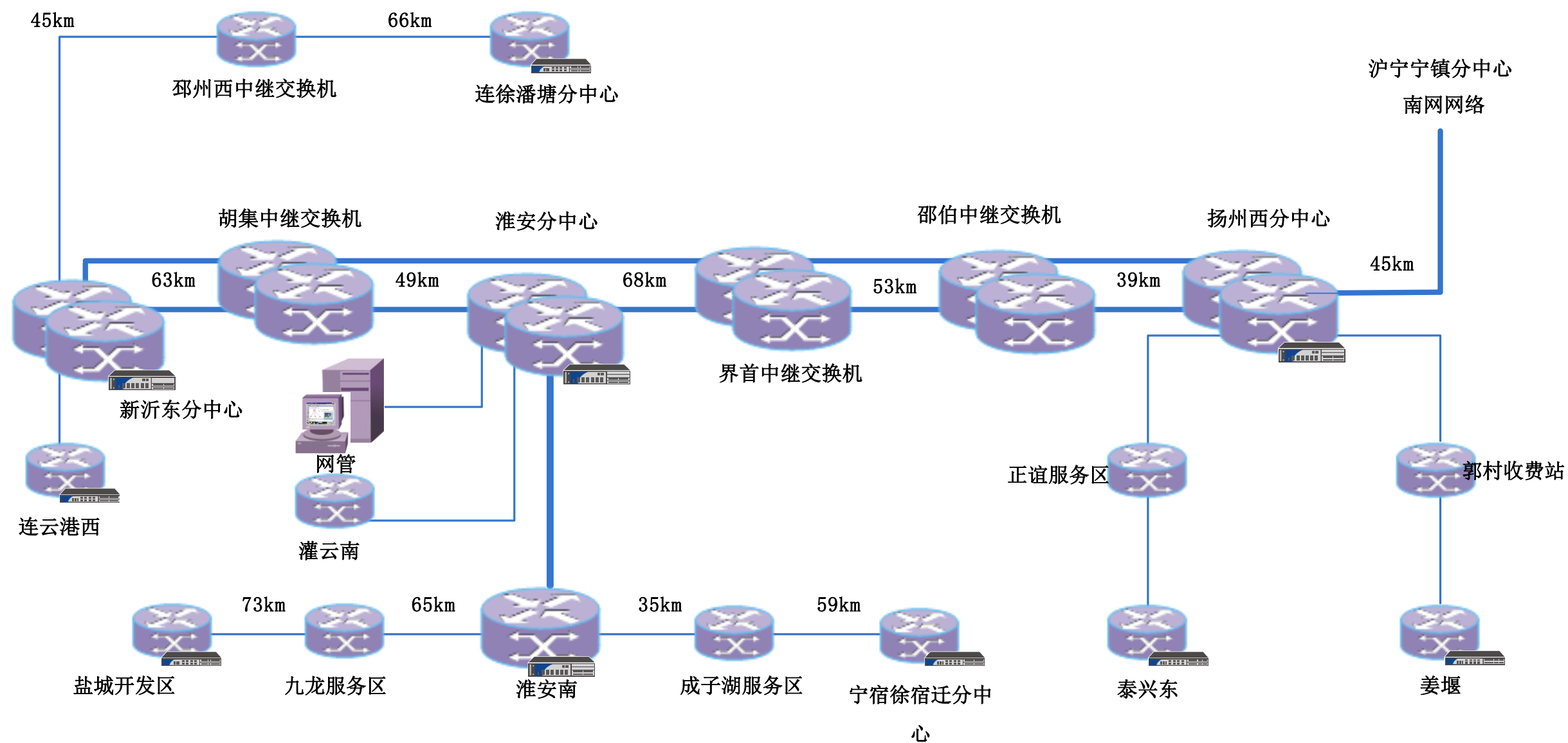
北网网络拓扑图
