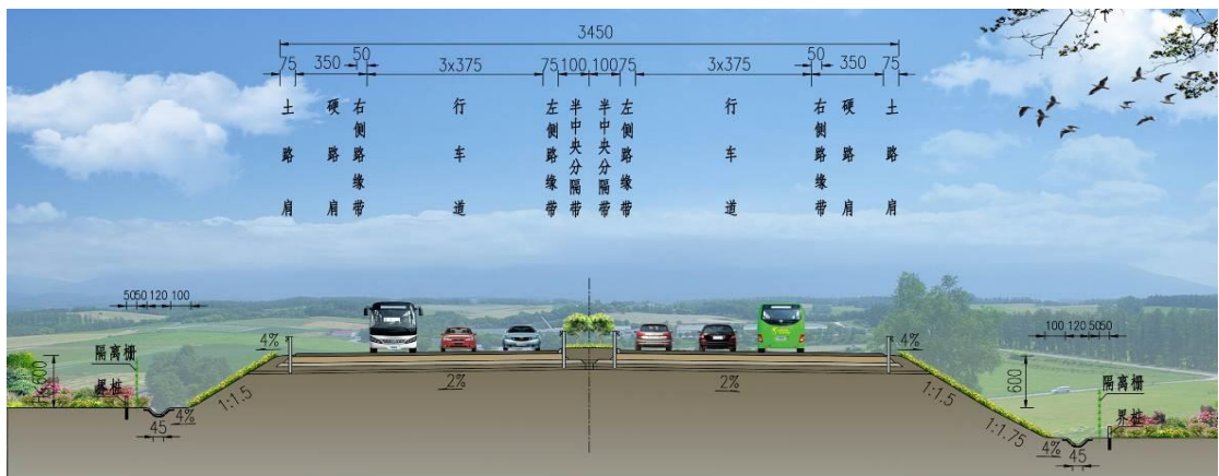
马山互通~南泉枢纽段路基标准横断面图
