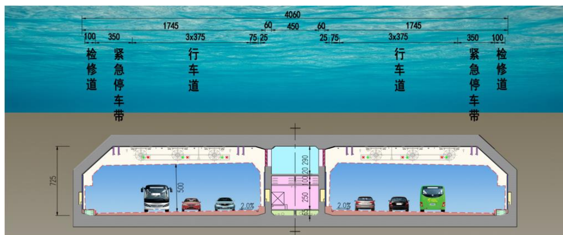
太湖隧道标准横断面图
