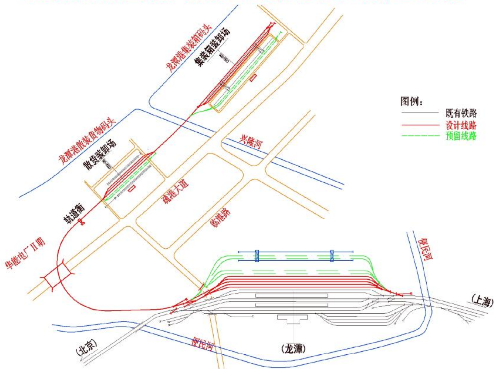
南京港龙潭港区铁路专用线可行性研究站场平面布置示意图
